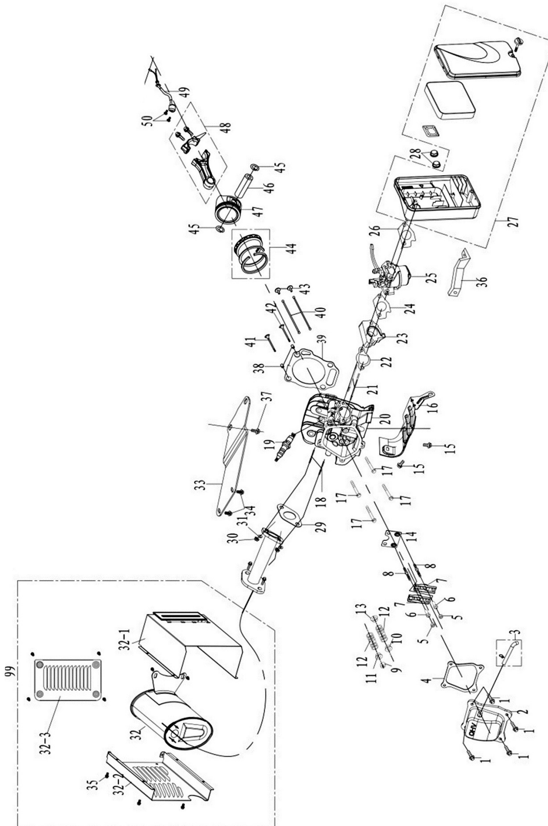
Abb. / Fig. 5: Ersatzteilzeichnung 5 / Spare parts drawing 5
