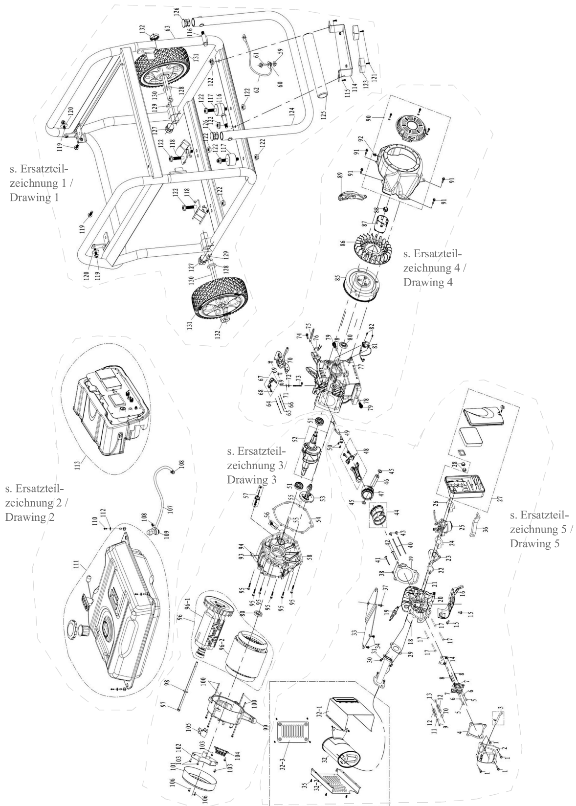
Abb. / Fig. 1: Gesamtansicht / General view
