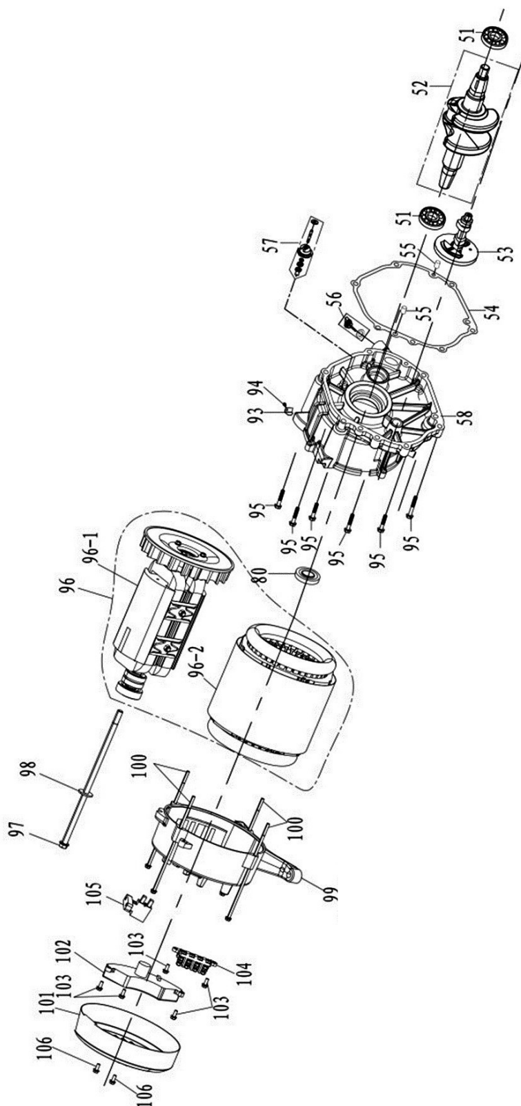
Abb. / Fig. 3: Ersatzteilzeichnung 3 / Spare parts drawing 3
