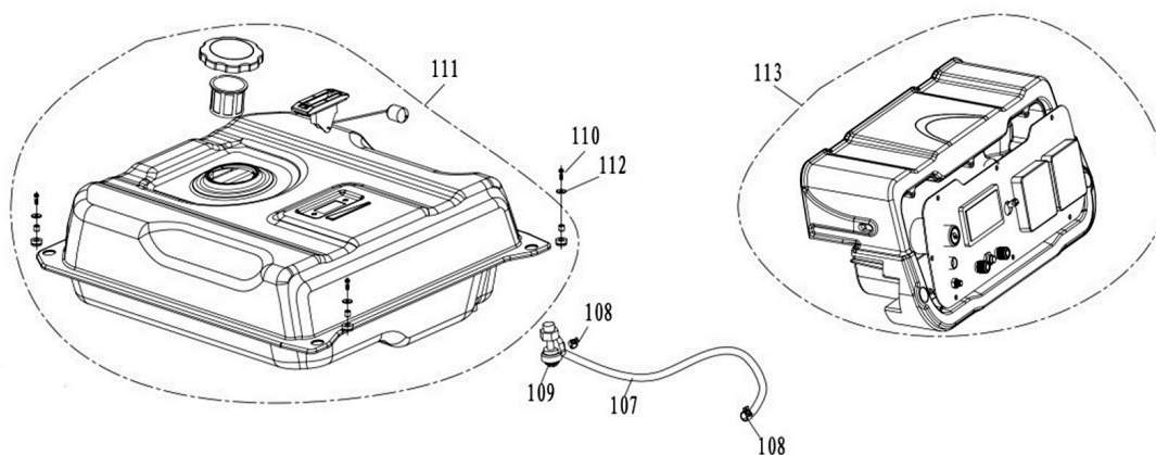
Abb. / Fig. 2: Ersatzteilzeichnung 1 & 2 / Spare parts drawing 1 & 2
