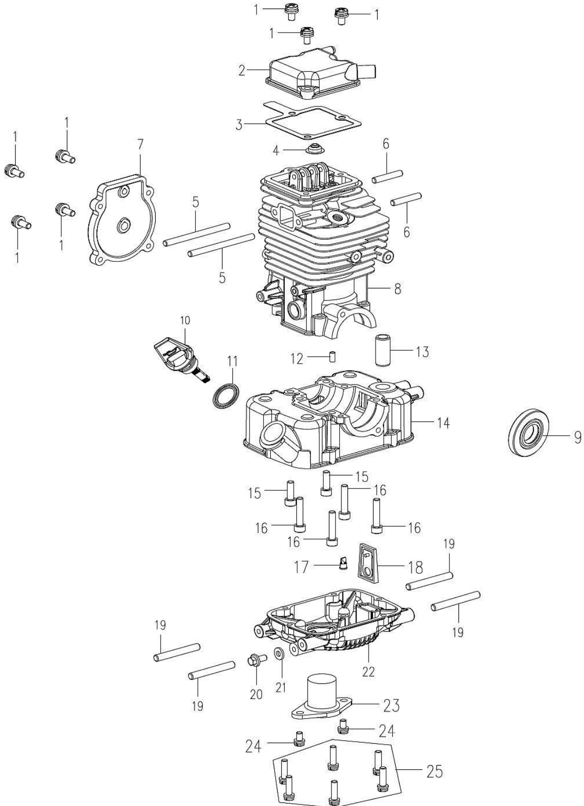
Abb. / Fig. 15: Ersatzteilzeichnung 1 / Spare parts drawing 1 PG-I 12 SR
