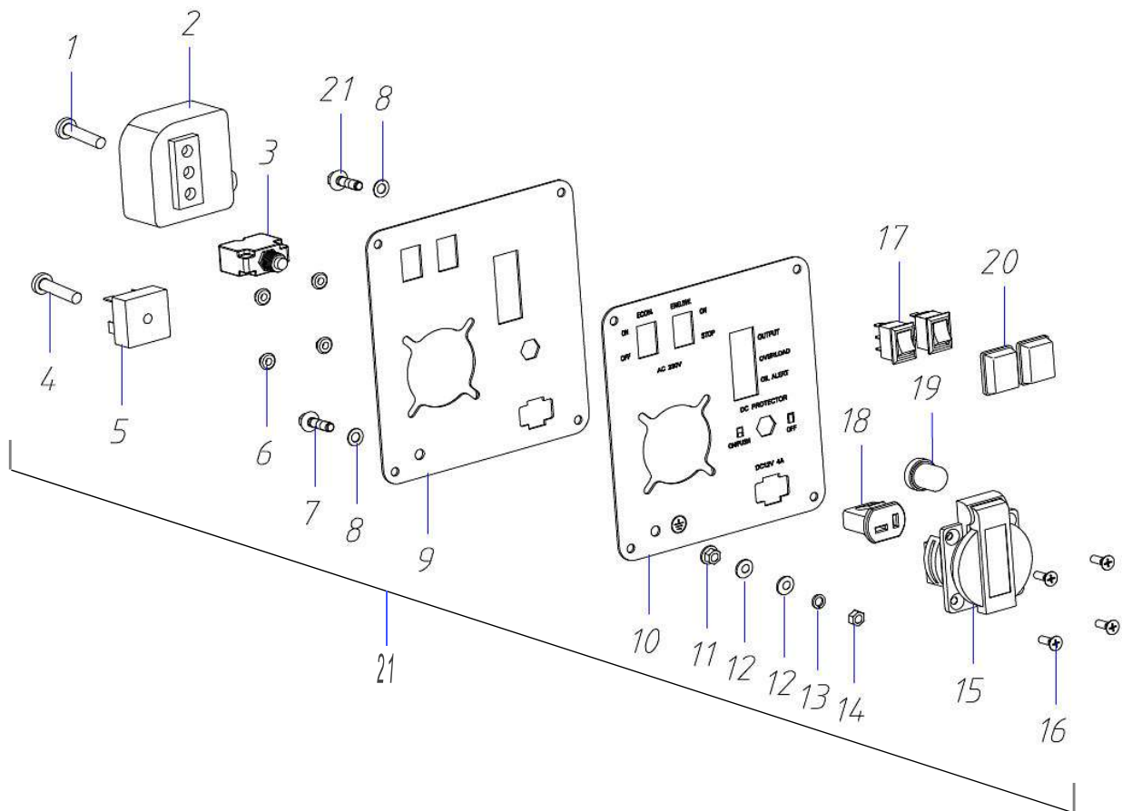
Abb. / Fig. 28: Ersatzteilzeichnung 14 / Spare parts drawing 14 PG-I 12 SR
