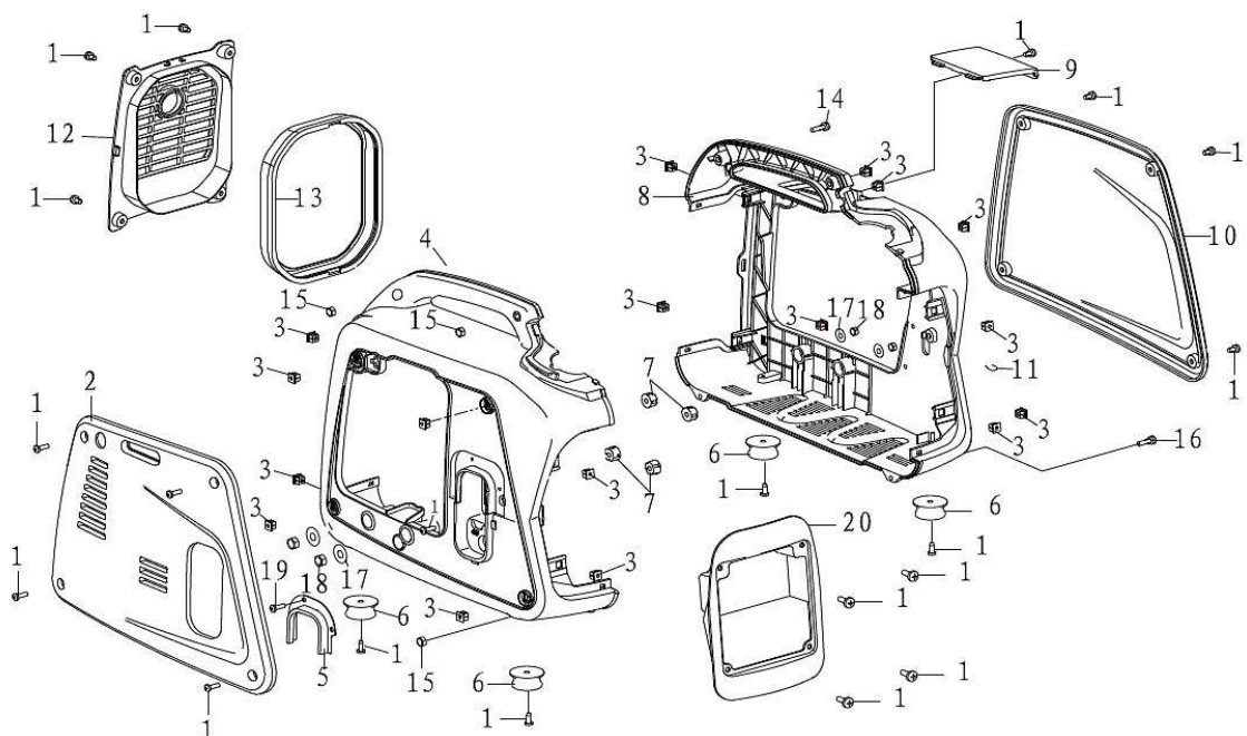
Abb. / Fig. 25: Ersatzteilzeichnung 11 / Spare parts drawing 11 PG-I 12 SR
