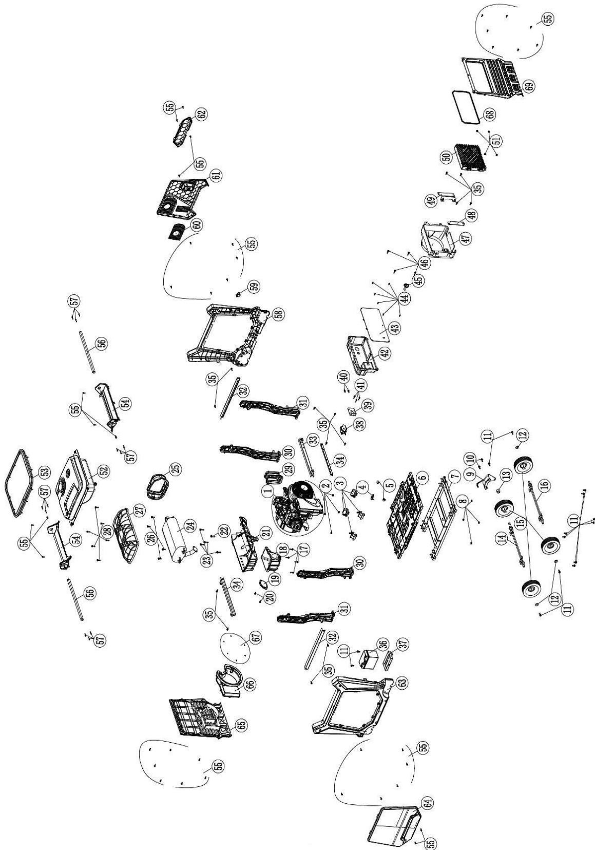
Abb. / Fig. 10: Ersatzteilzeichnung 1 PG-I 80 SE / Spare parts drawing 1 PG-I 80 SE
