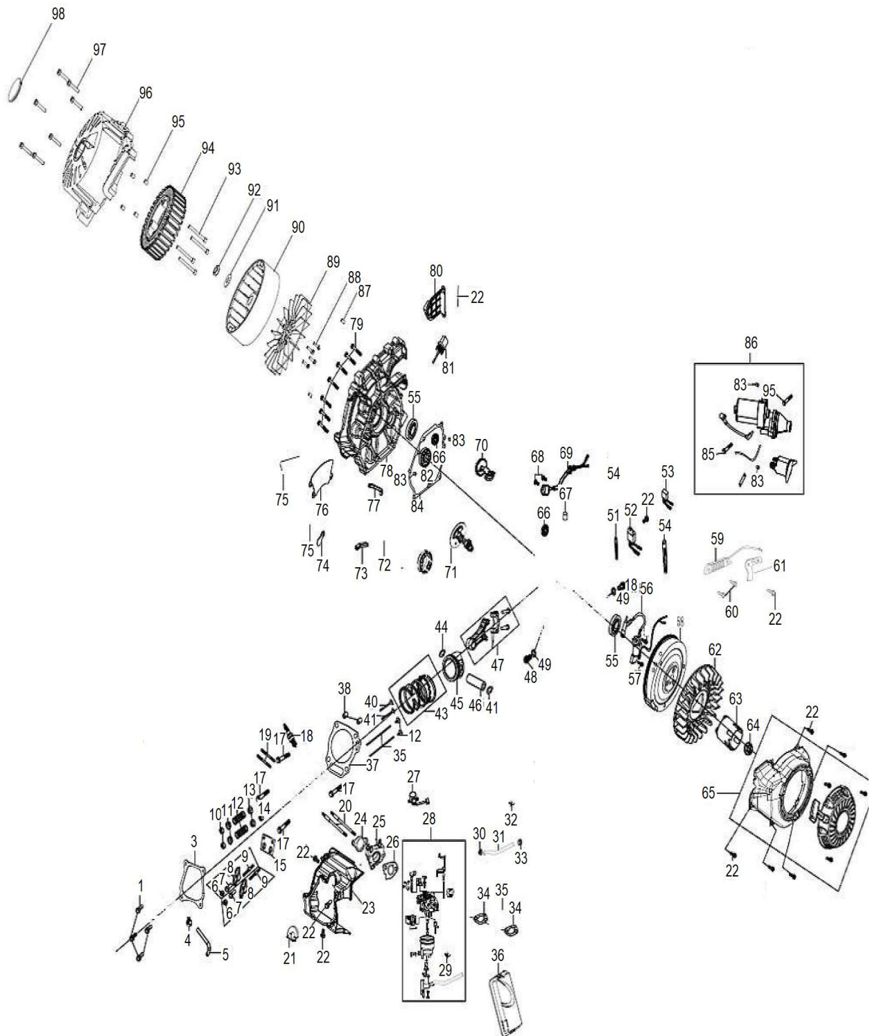
Abb. / Fig. 11: Ersatzteilzeichnung 2 PG-I 80 SE / Spare parts drawing 2 PG-I 80 SE
