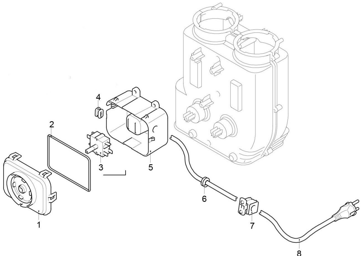
Abb. / Fig. 4: Ersatzteilzeichnung 4 und Ersatzteilzeichnung 5 / Spare parts drawing 4 and Spare parts drawing 5
