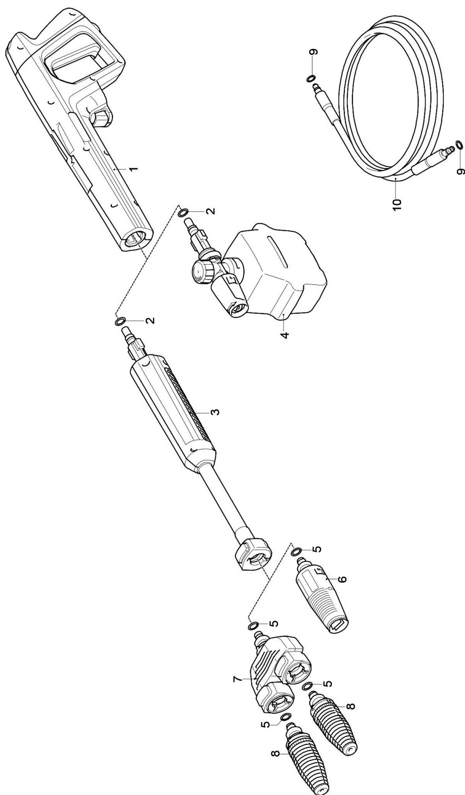
Abb. / Fig. 3: Ersatzteilzeichnung 3 / Spare parts drawing 3
