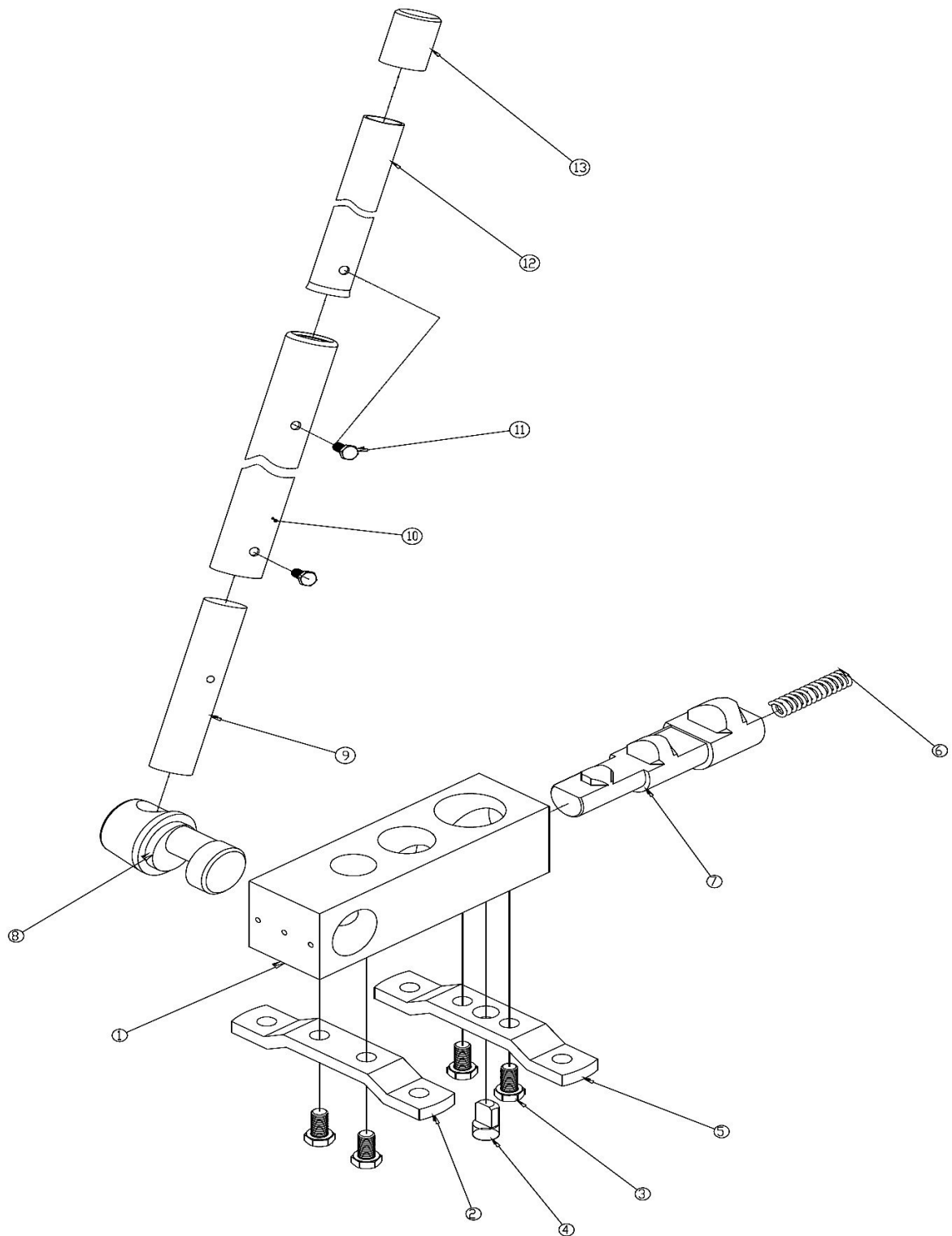
Abb. / Fig. 1: Ersatzteilzeichnung MRA 2 und MRA 3/ Spare parts drawing MRA 2 and MRA 3
