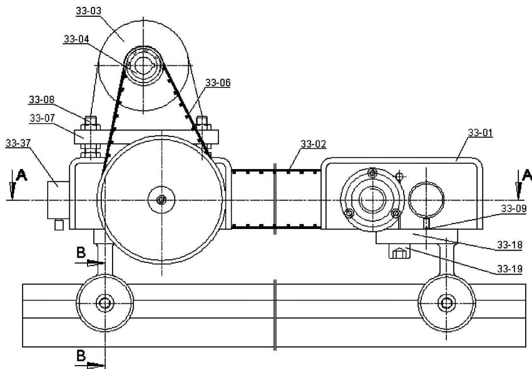
Abb. / Fig. 2: Ersatzteilzeichnung 2 / Spare parts drawing 2
