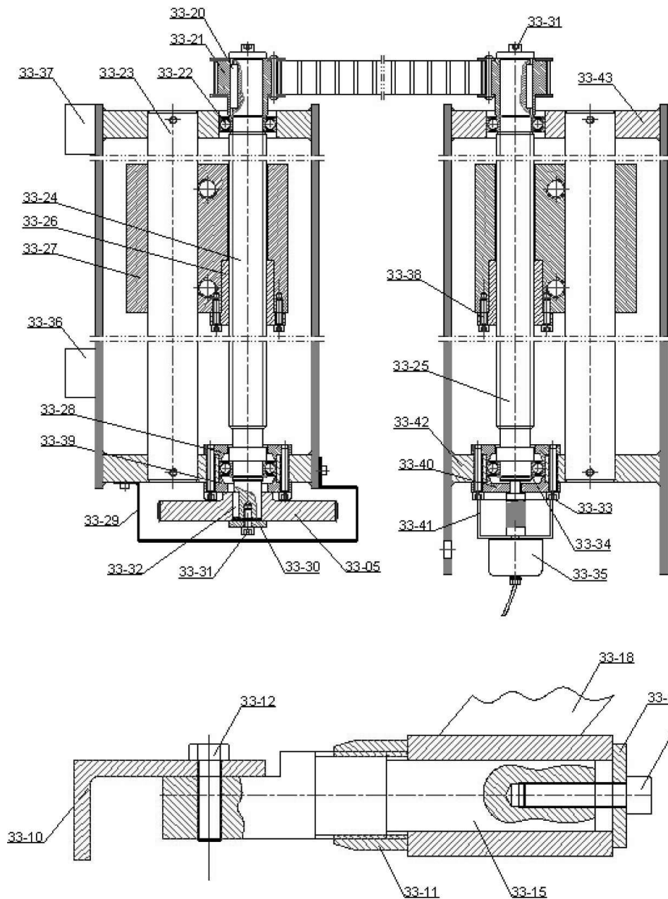
Ersatzteilzeichnung 3: Hinteranschlag, Teil 2 / Spare parts drawing 3: Backgauge, Part 2
