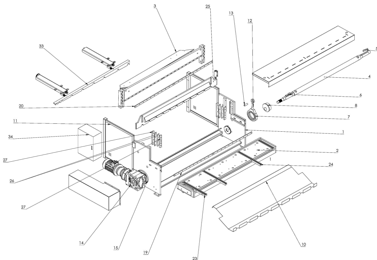
Abb. / Fig. 1: Ersatzteilzeichnung 1 / Spare parts drawing 1
