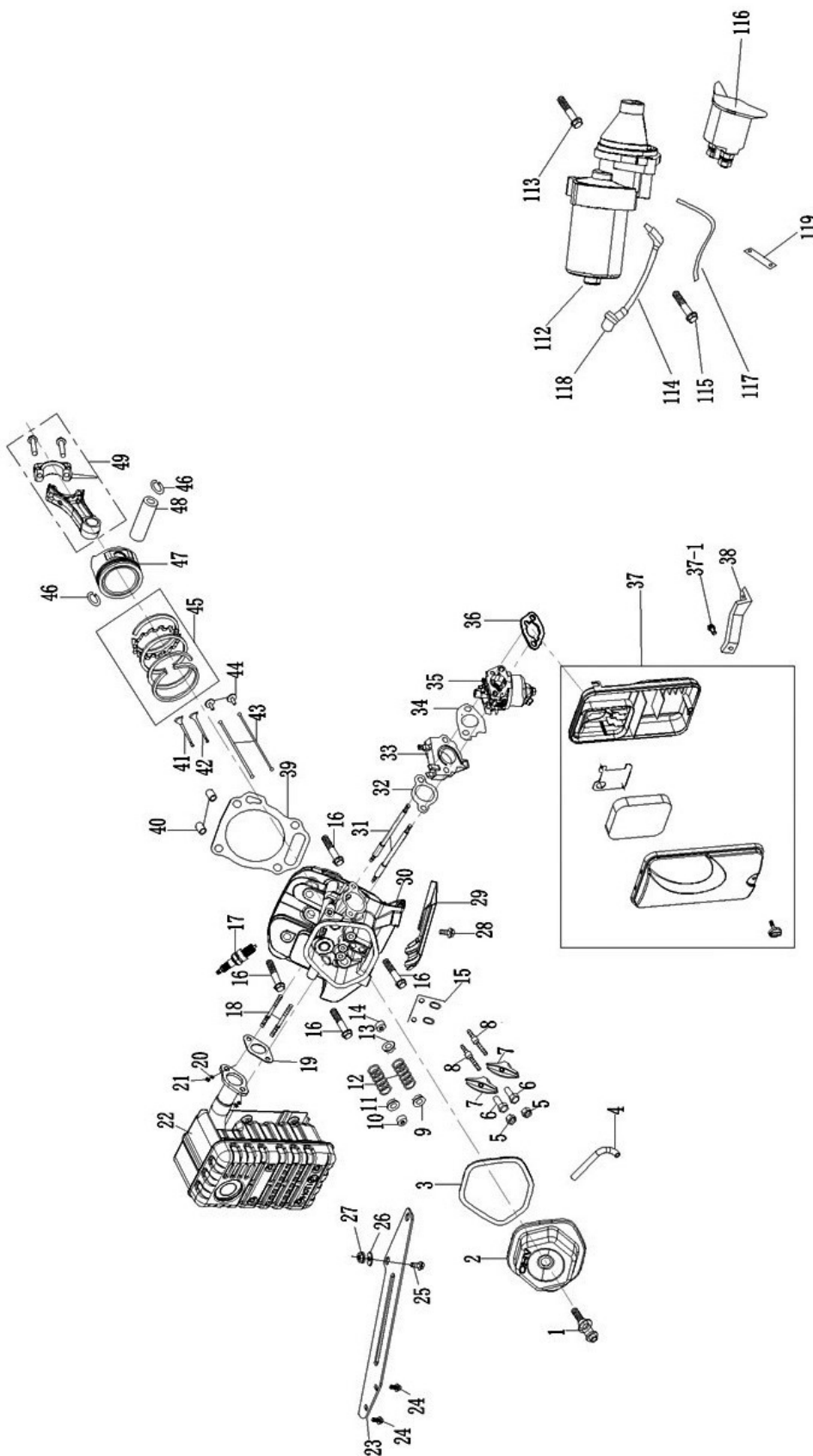
Abb. / Fig. 15: Ersatzteilzeichnung 5 / Spare parts drawing 5
