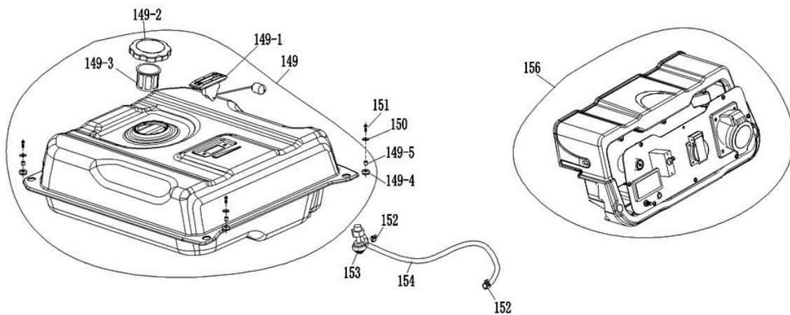
Abb. / Fig. 12: Ersatzteilzeichnung 1 & 2 / Spare parts drawing 1 & 2
