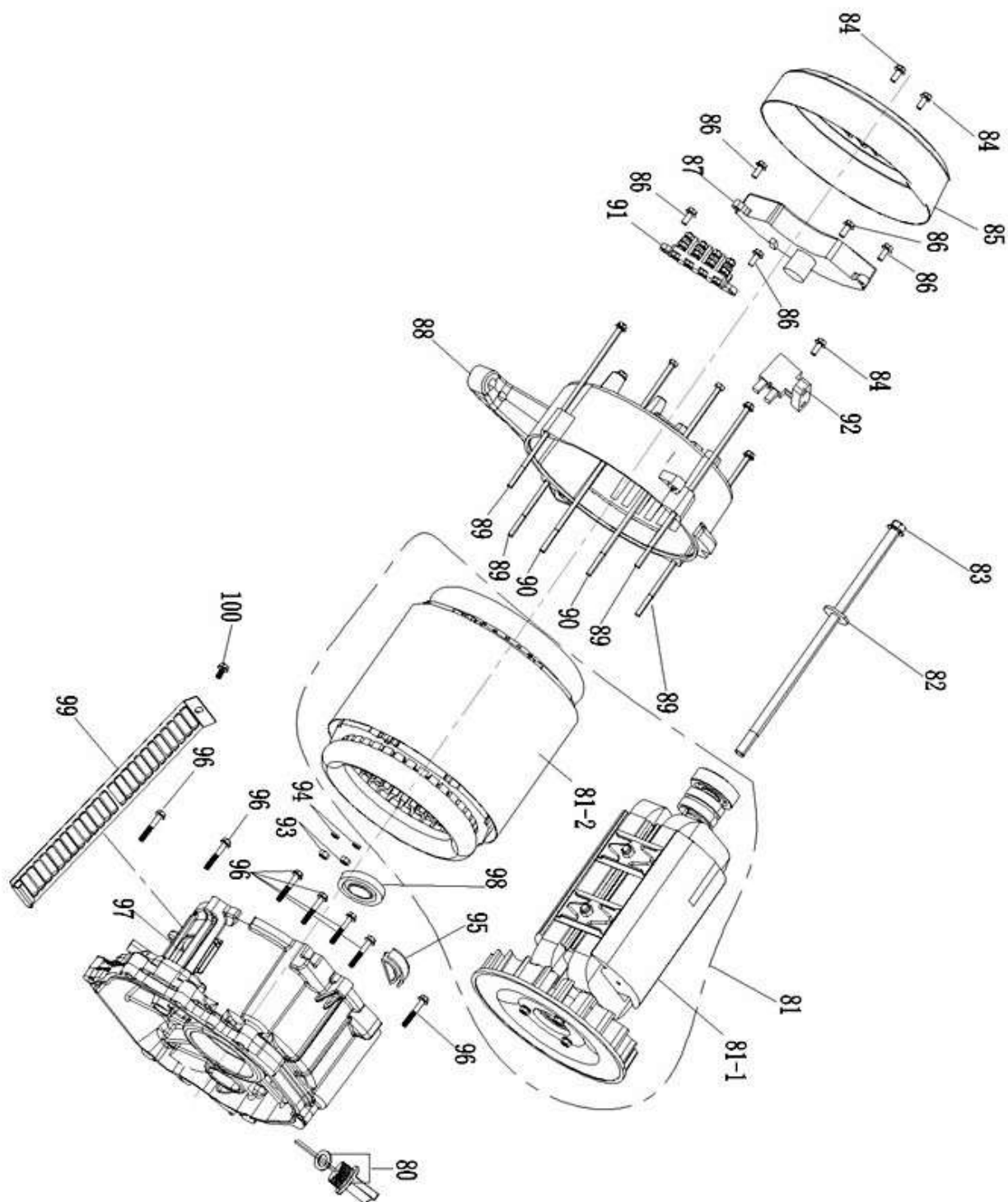
Abb. / Fig. 13: Ersatzteilzeichnung 3 / Spare parts drawing 3
