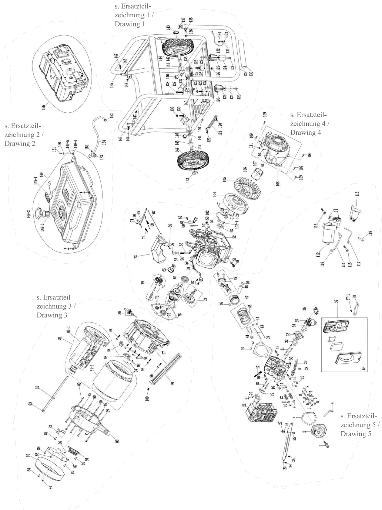
Abb. / Fig. 11: Gesamtansicht / General view PG-E 60 SEA & PG-E 80 TEA H
