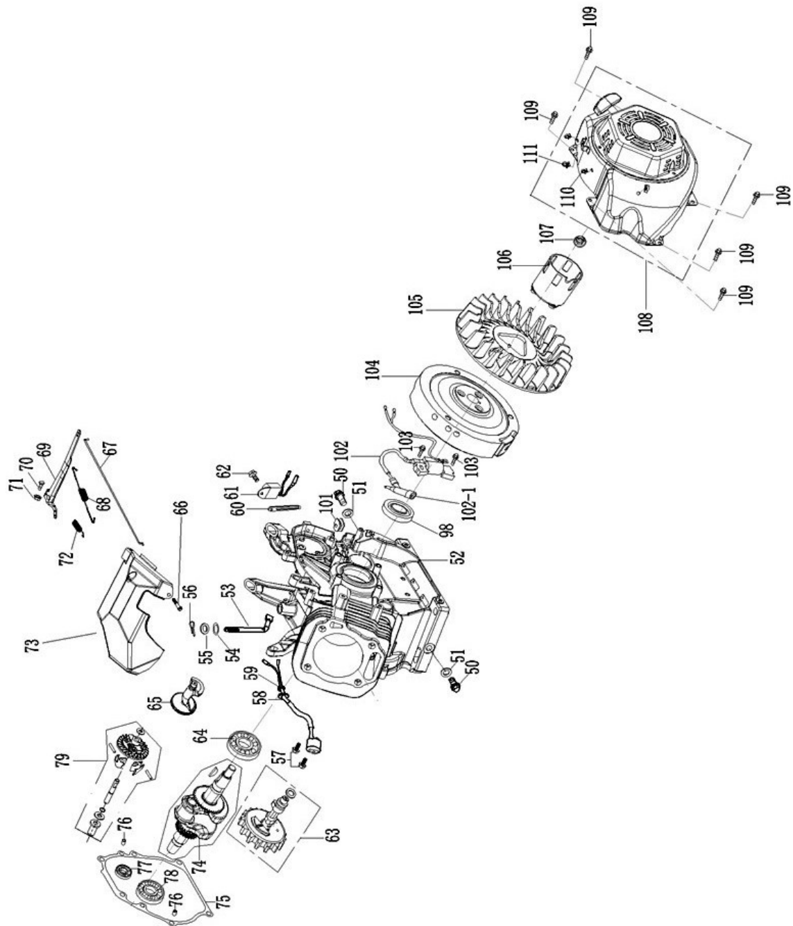
Abb. / Fig. 14: Ersatzteilzeichnung 4 / Spare parts drawing 4
